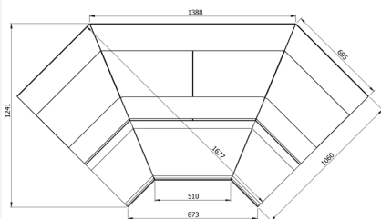
Vega S Corner IC 90
