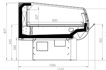
Vega S LG
